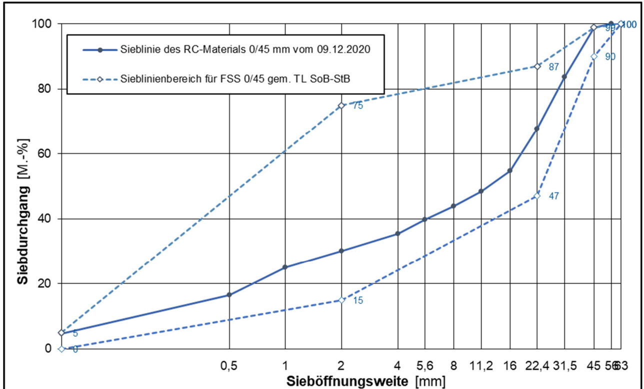
Korngrößenverteilung des untersuchten RC-Materials 0/45 mit Sieblinienbereich für Frostschuttschicht 0/45 mm gemäß TL SoB-StB /8/
