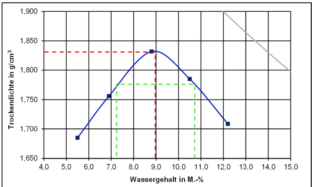
Proctorkurve des untersuchten RC-Materials 0/45 (aus Prüfbericht F 20/12/1231 – IV/2020)
