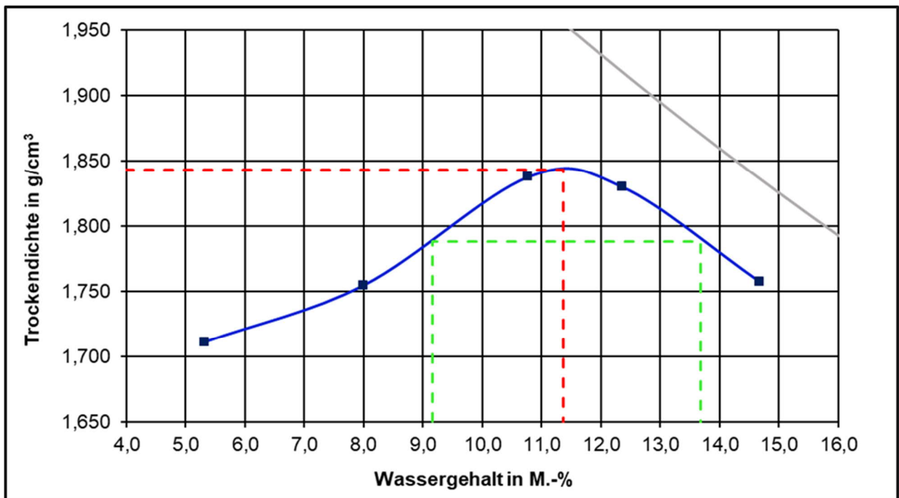
Proctorkurve des untersuchten RC Sand (aus Prüfbericht Nr. F 21/12/1154)
