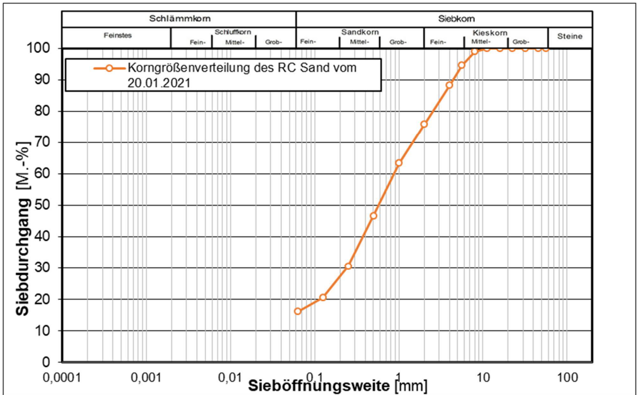
Korngrößenverteilung des untersuchten RC Sand
