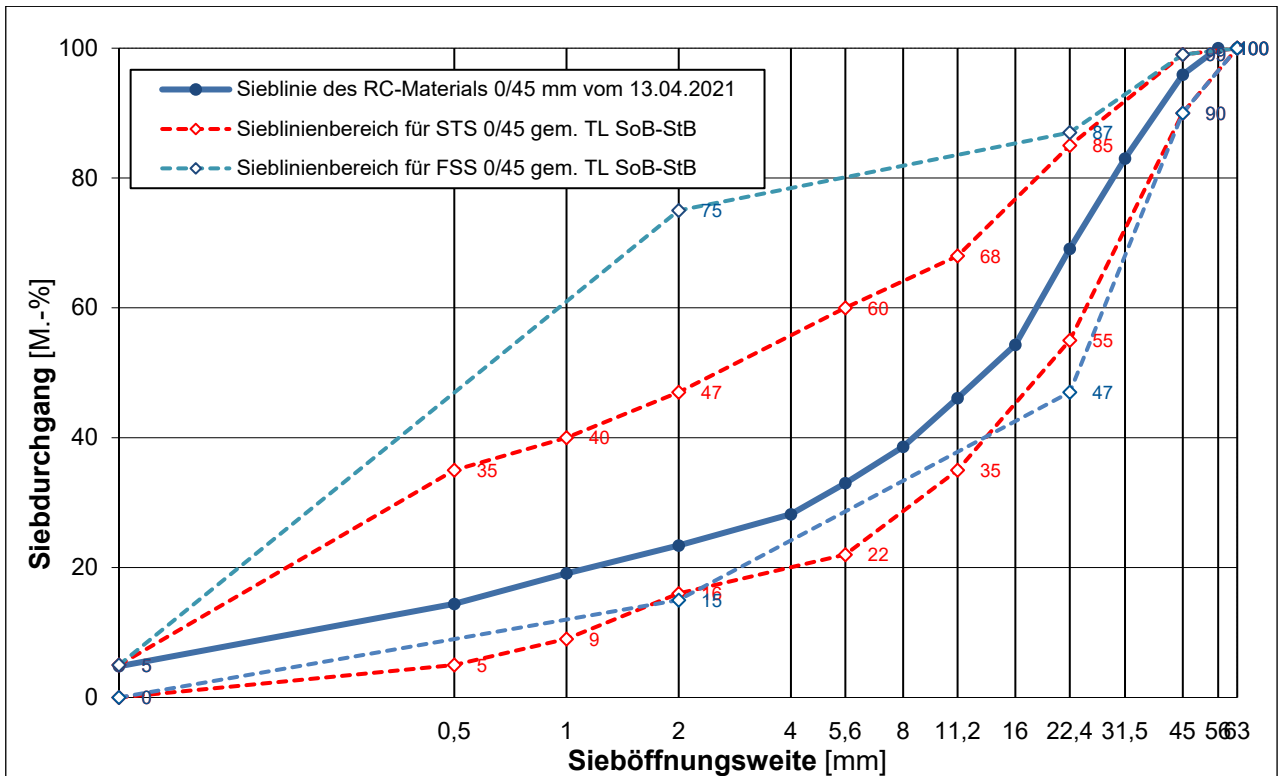
Korngrößenverteilung des untersuchten RC-Materials 0/45 mit Sieblinienbereich für Schottertrag- und Frostschuttschichten 0/45 mm gemäß TL SoB-StB /8/
