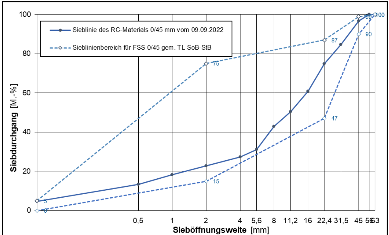
Korngrößenverteilung des untersuchten RC-Materials 0/45 mm mit Sieblinienbereich für Frostschuttschicht 0/45 mm gemäß TL SoB-StB /8/
