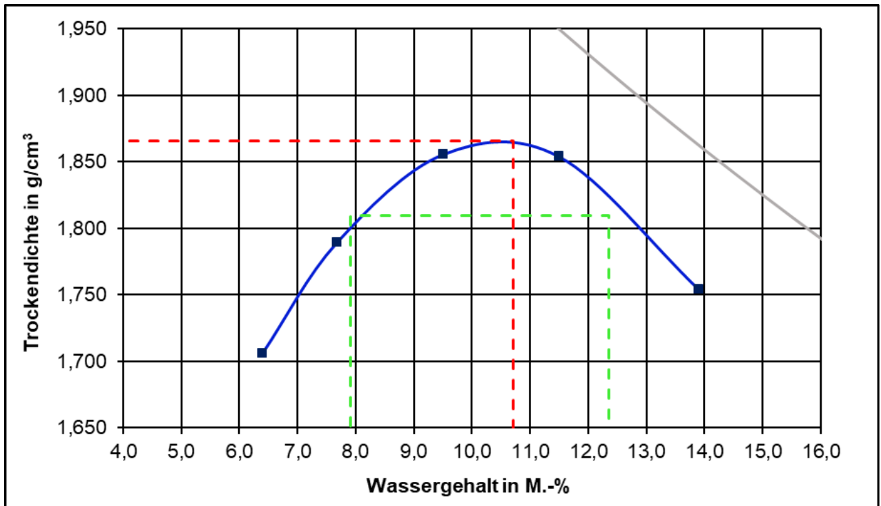
Proctorkurve des untersuchten RC-Materials 0/45 (aus Prüfbericht F 24/01/0114 B)
