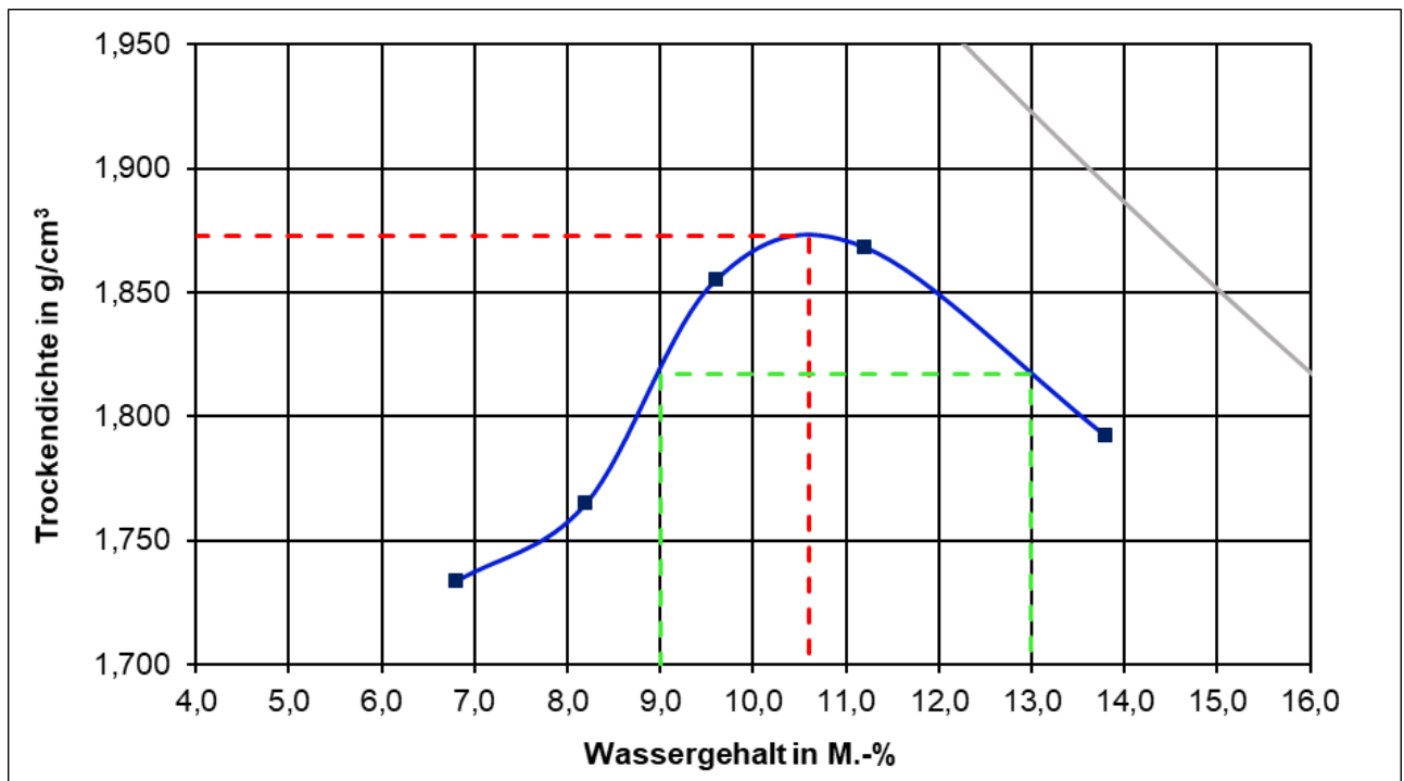
Proctorkurve des untersuchten RC-Materials 0/45 (aus Prüfbericht F 25/06/0593 B)
