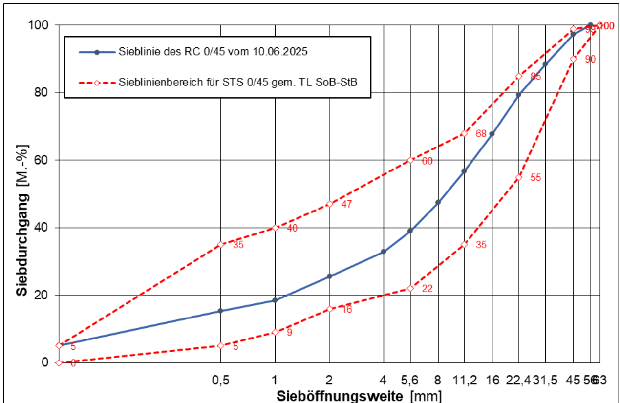
Korngrößenverteilung des untersuchten RC-Materials 0/45 mit Sieblinienbereich für Schottertragschicht 0/45 mm gemäß TL SoB-StB /8/
