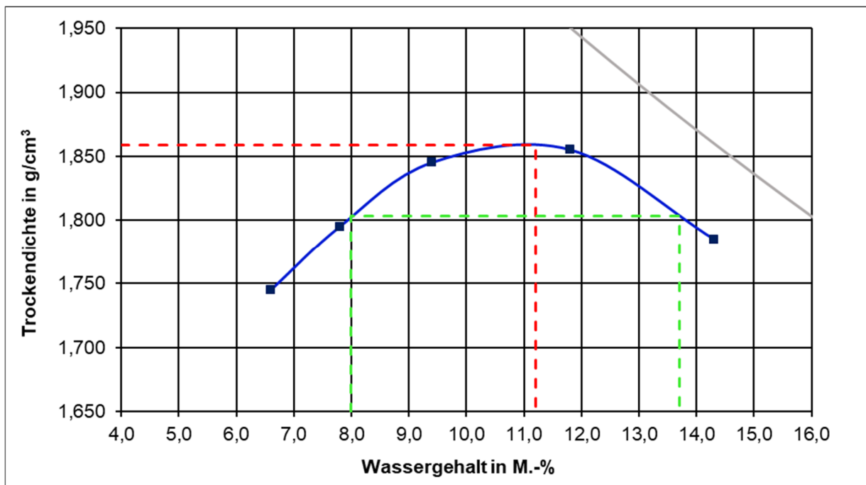
Proctorkurve des untersuchten RC Sand (aus KM Prüfbericht F 25/06/0594)
