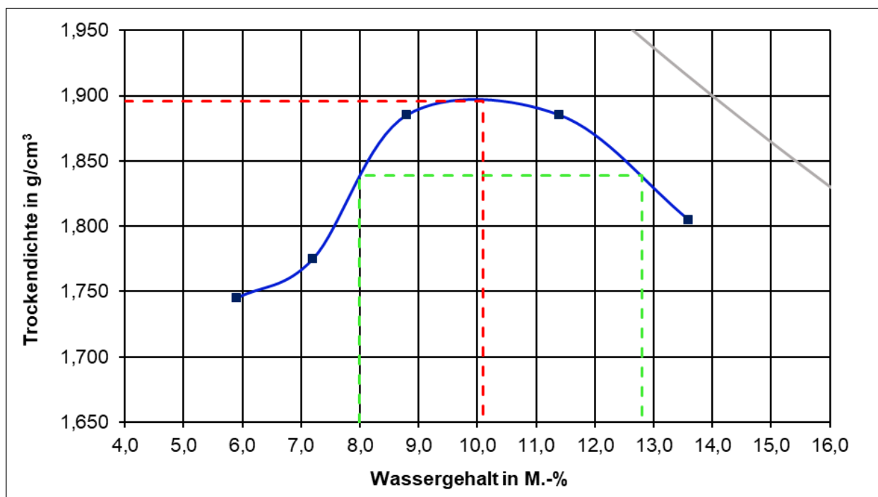
Proctorkurve des untersuchten RC-Materials 0/45 (aus Prüfbericht F 25/11/1359 B)
